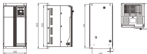
VH1-4018/4022-B
