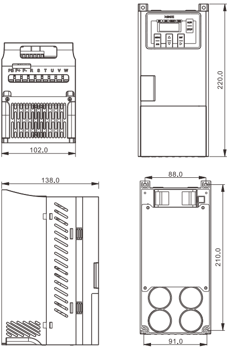
VH5-45P5-B
