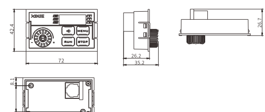
VH1-PE100
