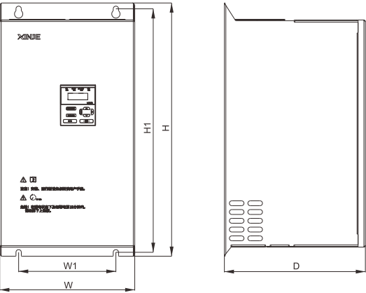
VH-P4110
