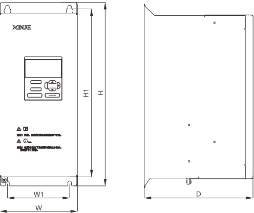
VH-P4030
