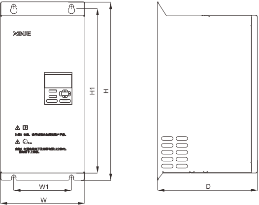
VH-P4055
