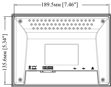
Вид сзади
