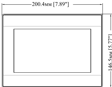
Вид спереди
